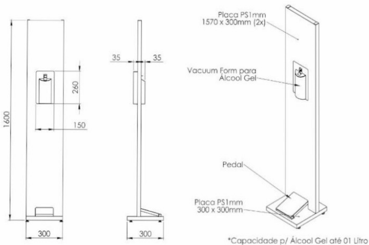
Figura 1 – Especificações do Totem de Álcool Gel
