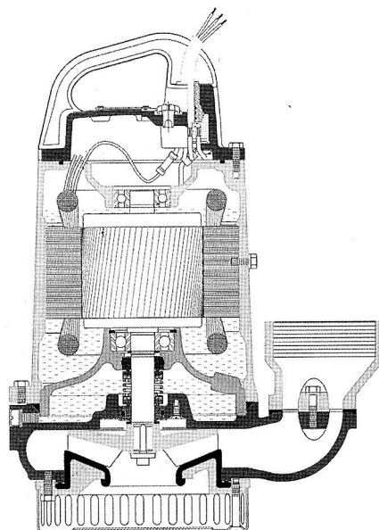
Imagem em corte de uma UNI 1000T
