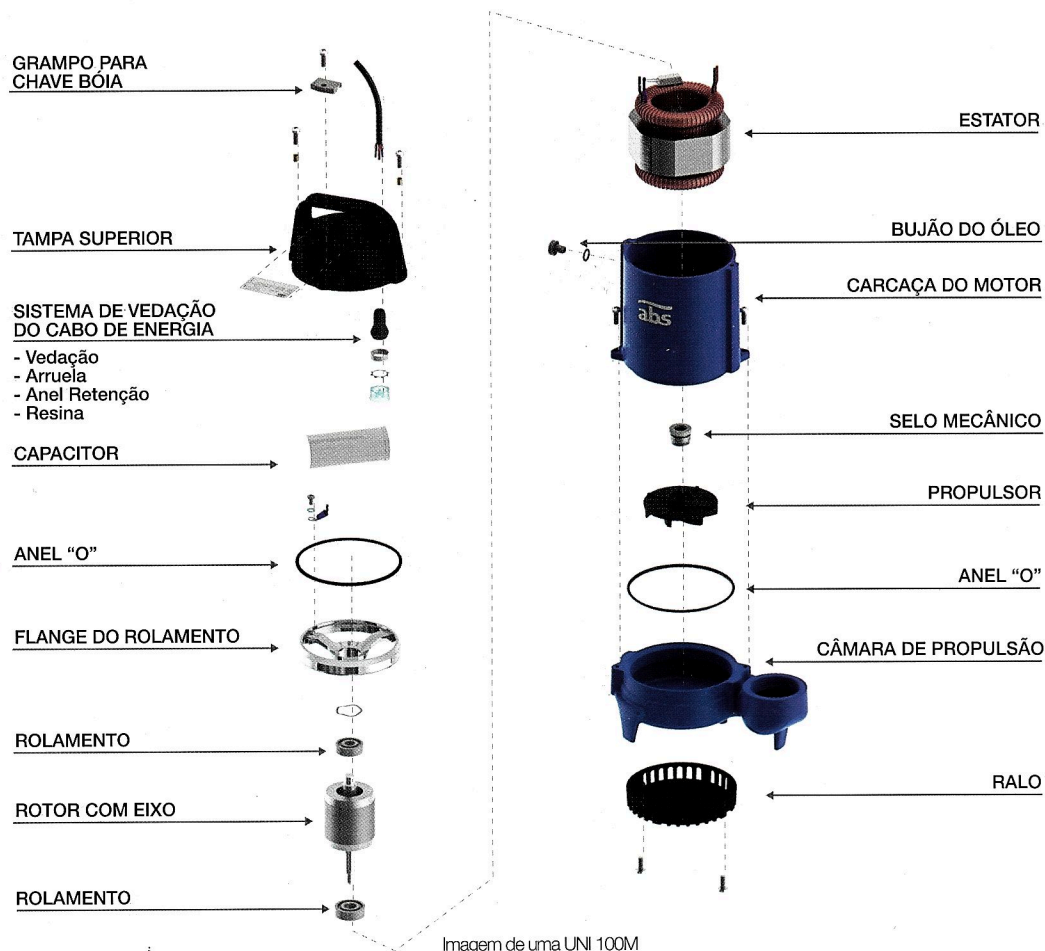
Imagem de uma UNI 100M
