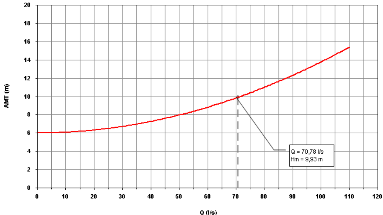
CURVA DO SISTEMA - ESTAÇÃO ELEVATÓRIA EE-39
