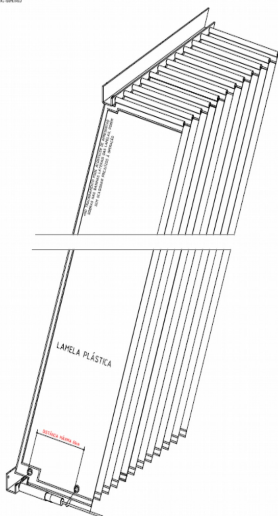
FIXAÇÃO DA LAMELA PLÁSTICA DISPOSIÇÃO GERAL – ISOMÉTRICO SEM ESCALA
