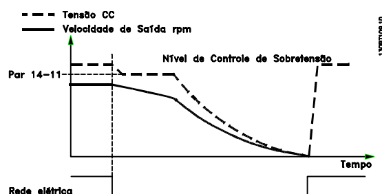
Ilustração 2.5: Back-up Cinético, falha mais longa da rede elétrica. O motor é parado por inércia tão logo a energia no sistema esteja muito baixa.
