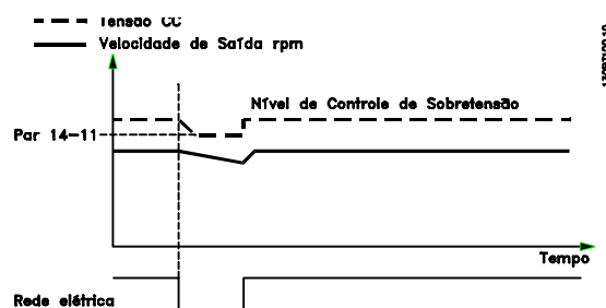
Ilustração 2.4: Back-up Cinético, falha de curta duração da rede elétrica. Prossiga enquanto a energia no sistema permiti-lo.
