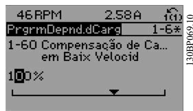
Ilustração 1.17: Exemplo de display
