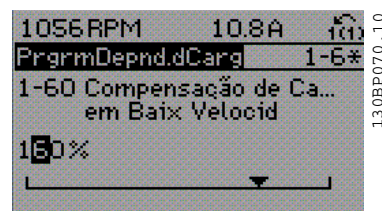
Ilustração 1.18: Exemplo de display.
