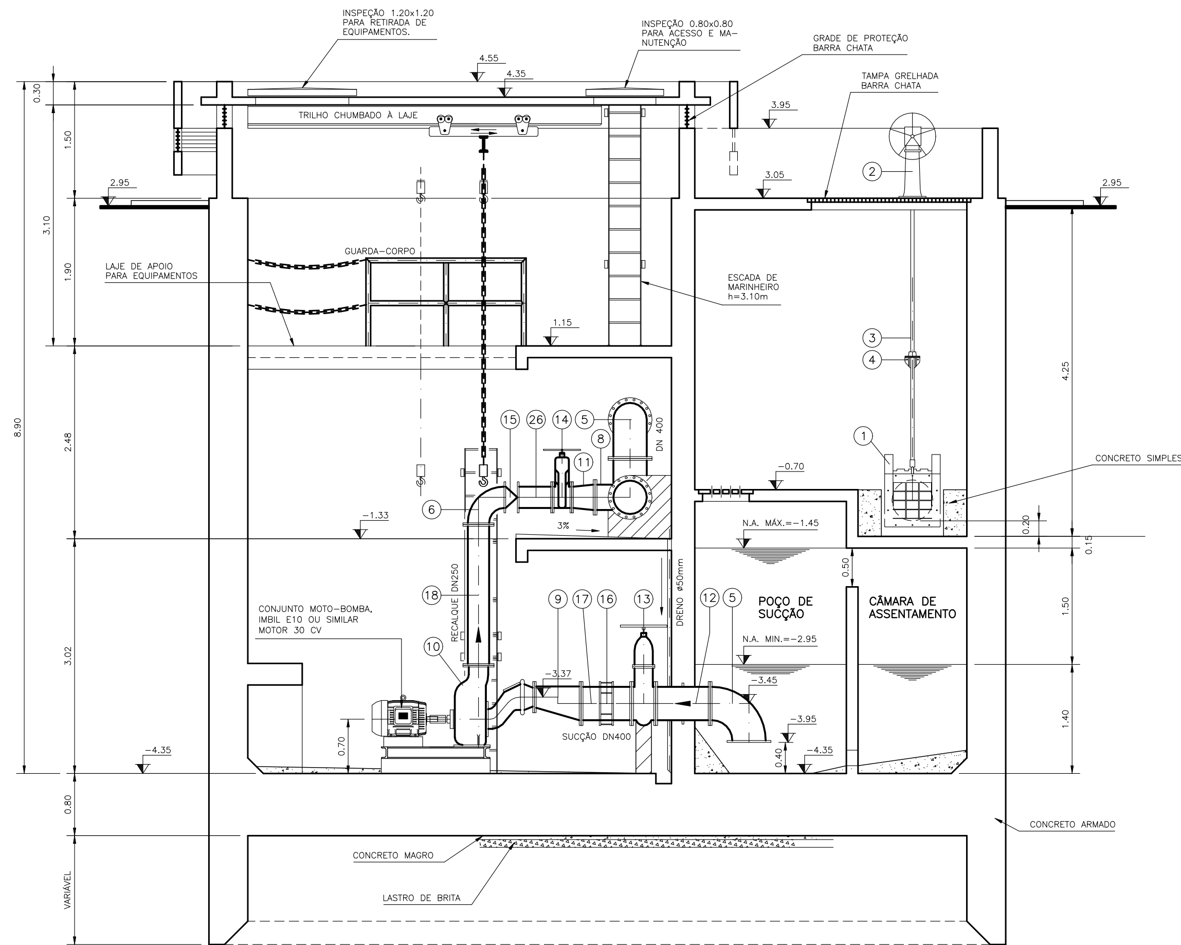
CORTE A-A
