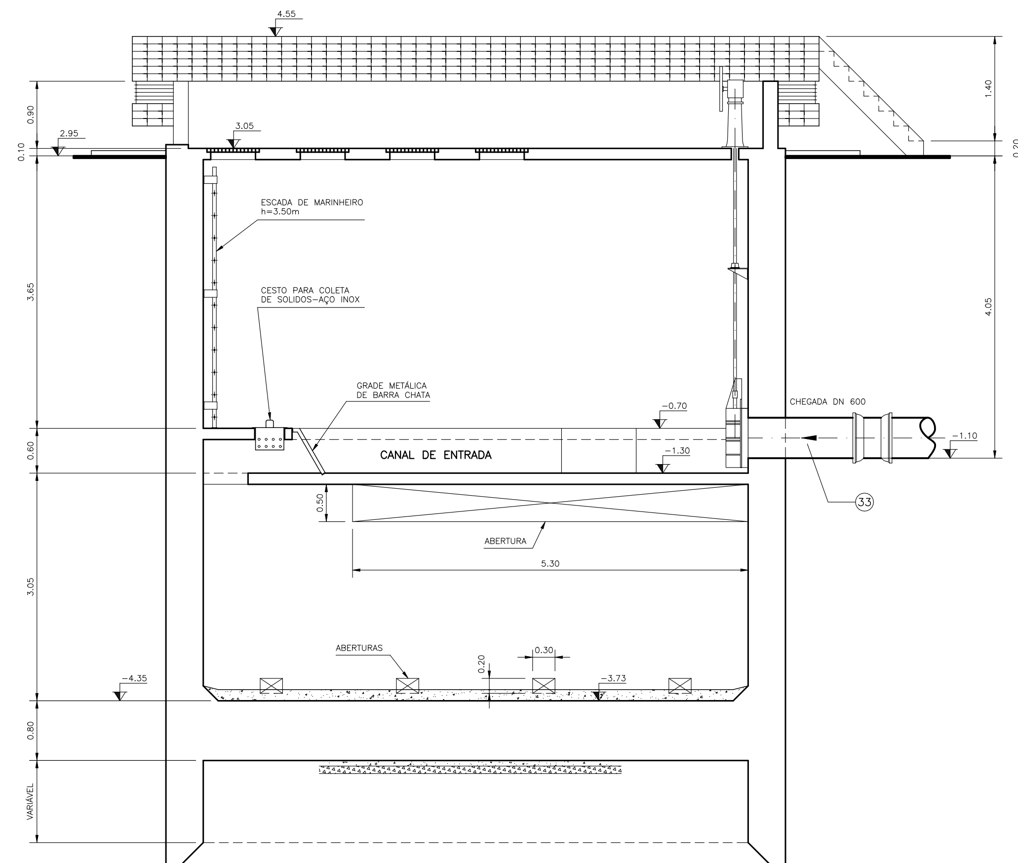
CORTE C-C
