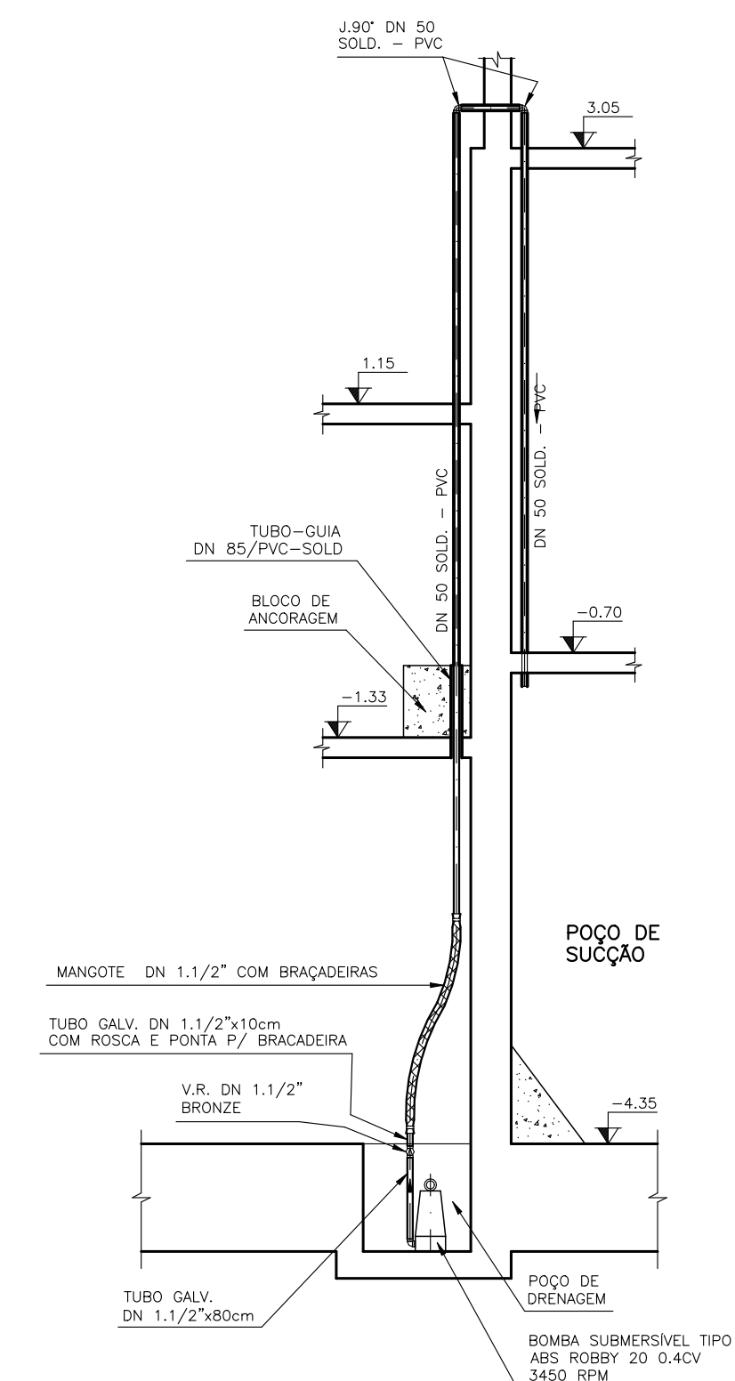
CORTE D-D
