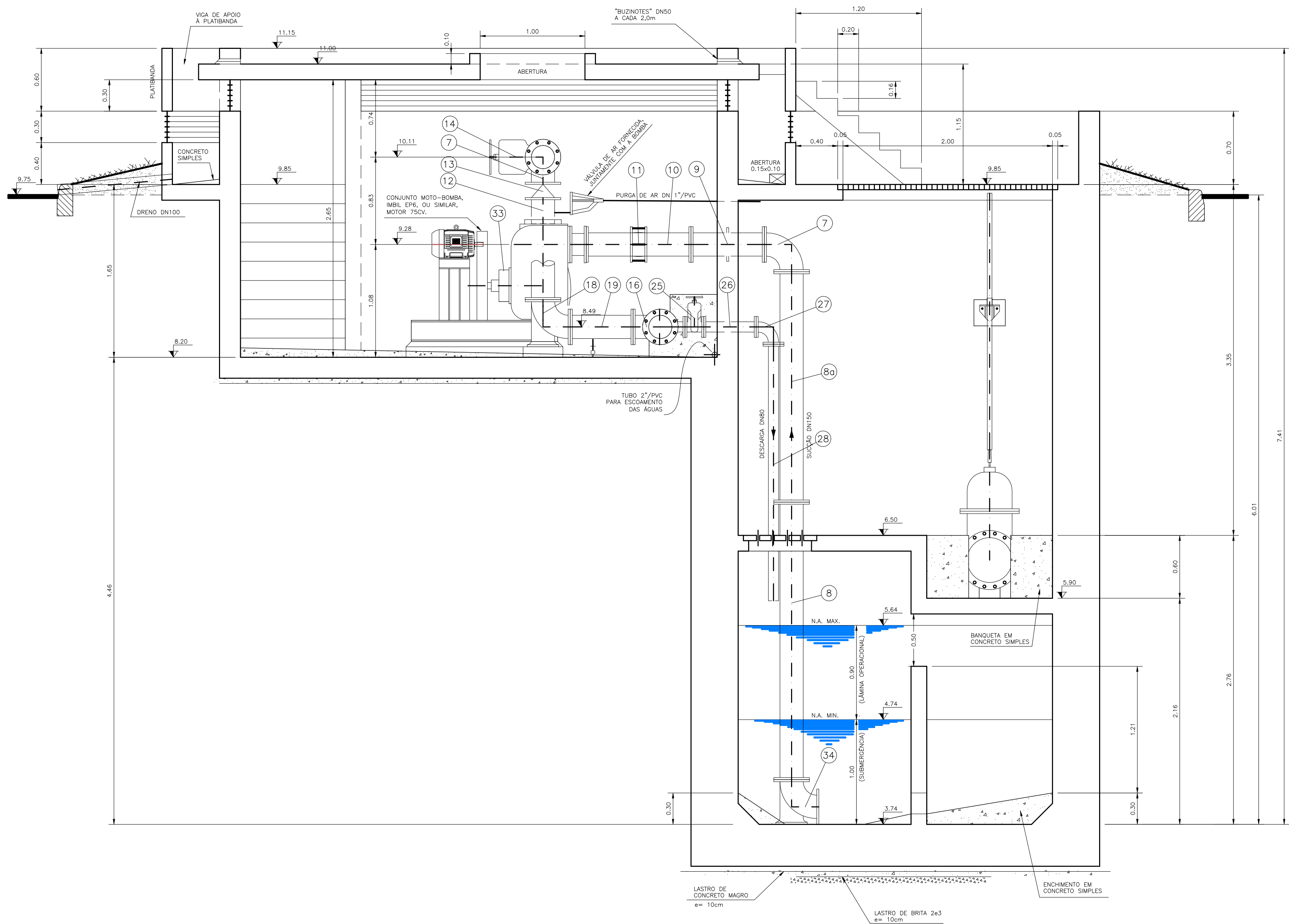
CORTE C-C ESC. 1:25
