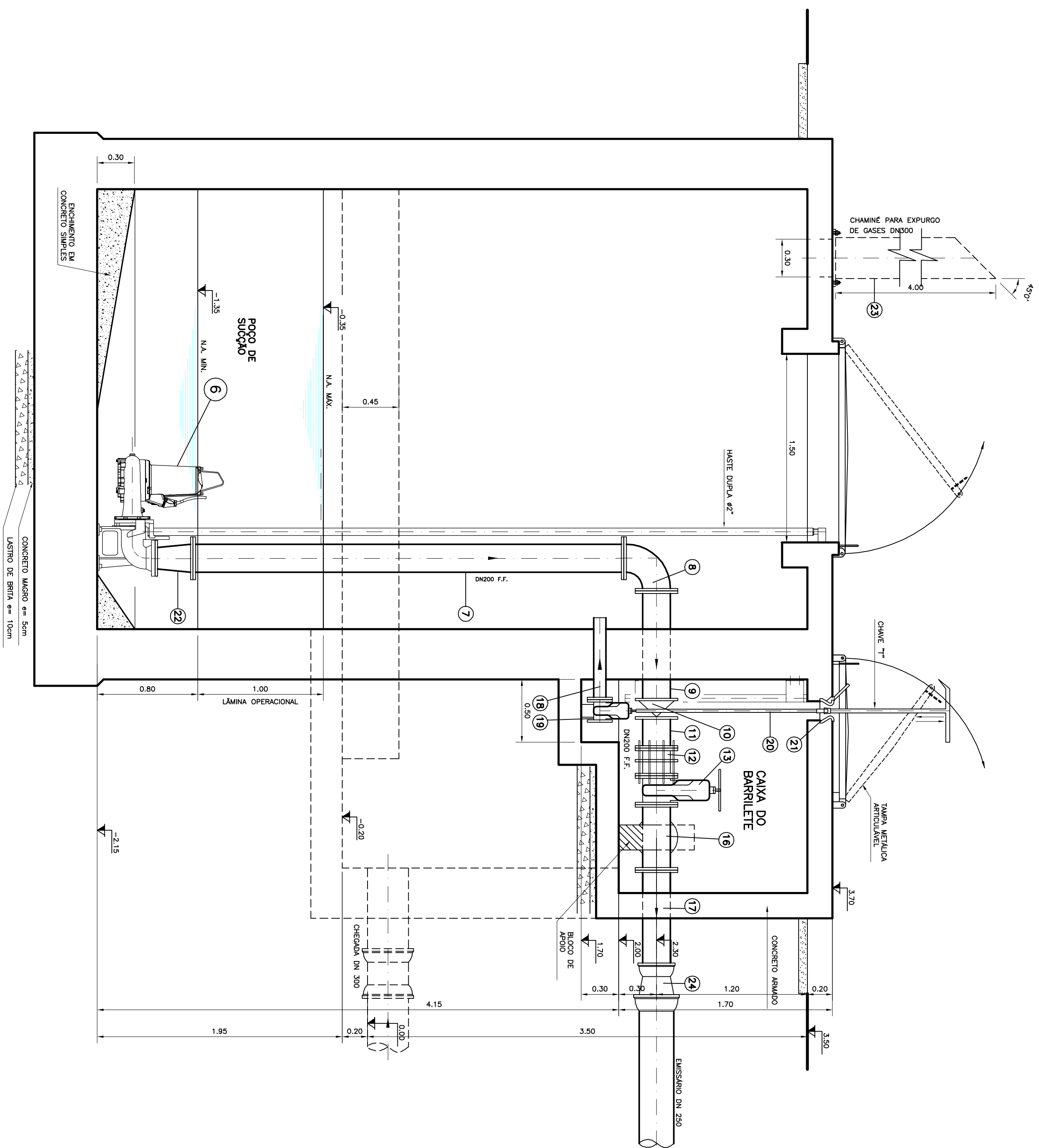
CORTE A-A ESC. 1:25
