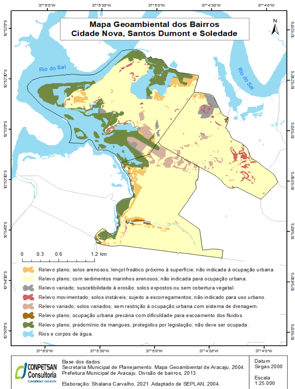
Figura 31 - Mapa Geoambiental dos bairros Cidade Nova, Santos Dumont e Soledade.
