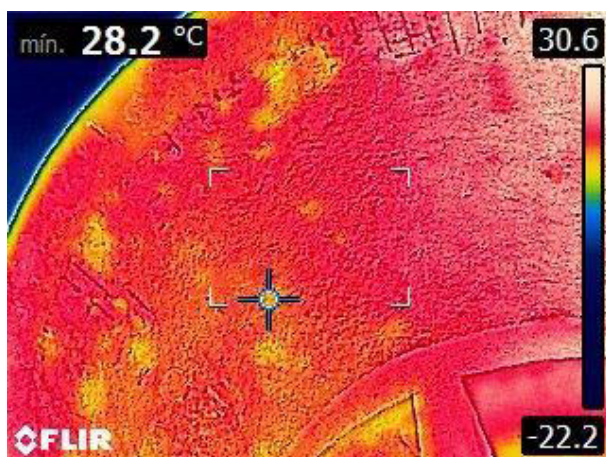
Figura 43 – Ensaio de termografia executado na parede da cuba inferior com visualização de pontos de umidade e vazamento.
