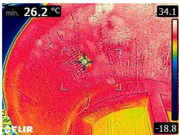
Figura 39 – Ensaio de termografia executado na parede da cuba inferior com visualização de pontos de umidade e vazamento.
