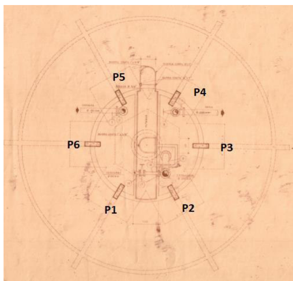
Figura 25 – Planta baixa do reservatório.
