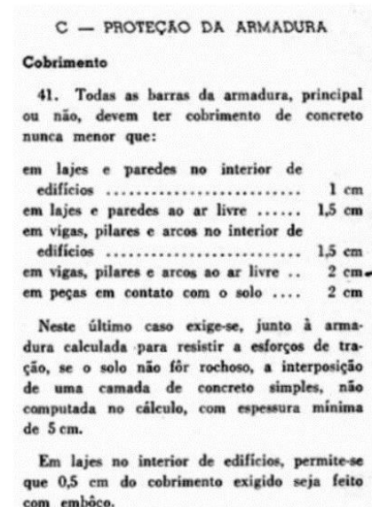
Figura 30 – Espessura dos cobrimentos segundo a NB-1/60
