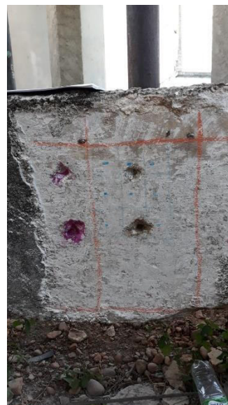
Figura 34 – Resultado do ensaio de Carbonatação na viga V1
