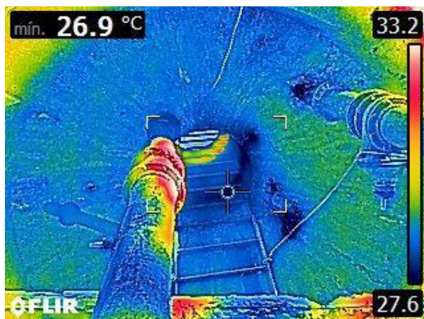
Figura 47 – Ensaio de termografia executado no fundo com visualização de pontos de umidade e vazamento.
