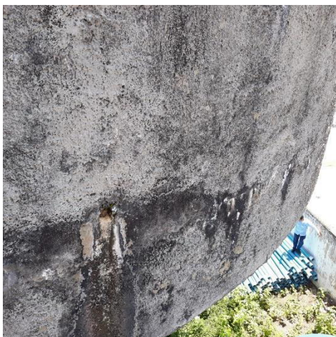
Figura 56 – Parede do reservatório com vazamento pelas juntas.
