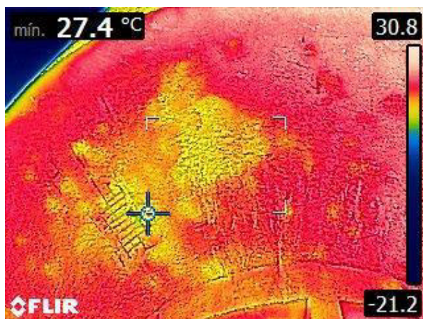
Figura 45 – Ensaio de termografia executado na parede da cuba inferior com visualização de pontos de umidade e vazamento.
