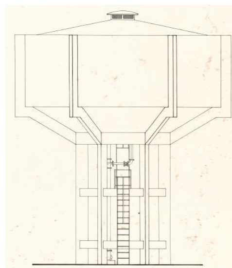
Figura 26 – Vista do reservatório.
